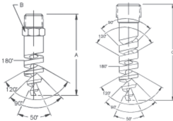
罐子清洗 XGLX 覆盖表 喷雾压力为 2 到 3 巴
